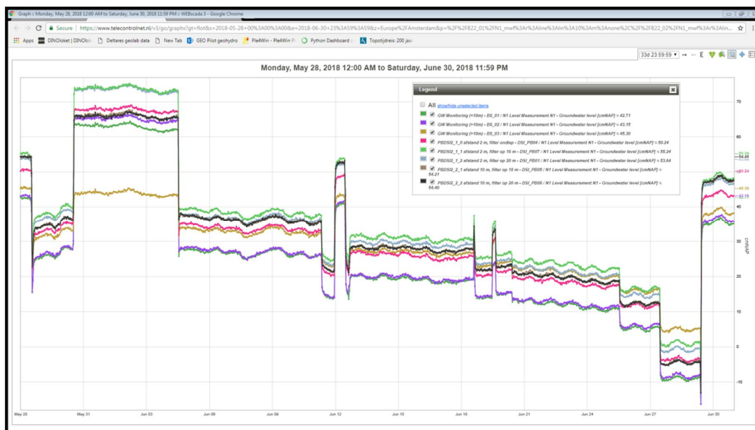
Figuur 10.5 Stijghoogteverandering bij DSI-streng 2 achter de zuivering. Retour op streng 2 was van 30 mei tot 4 juni 12:00. Effecten daarna zijn het gevolg van pompen uit PP2 en retour op DSI-streng 1 in retourveld
